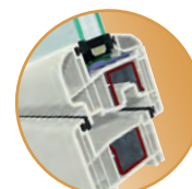
σύστημα 6 θαλάμων Ημι-μετατοπισμένο πλαίσιο
